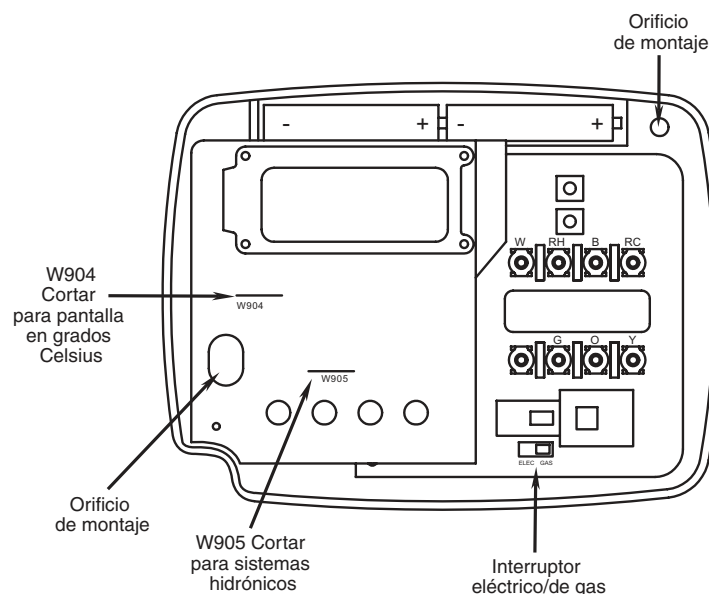
Figura 1. Base del termostato
