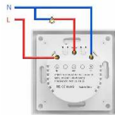
SCHÉMA ZAPOJENÍ
